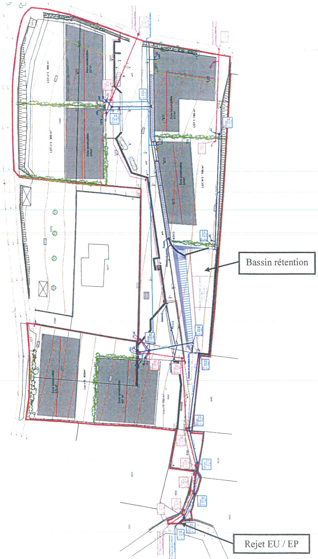
Figure n°12 : Schéma des réseaux d'assainissement
